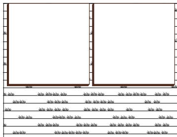
POSA A SECCO SU ERBA DRY LAYING ON GRASS
