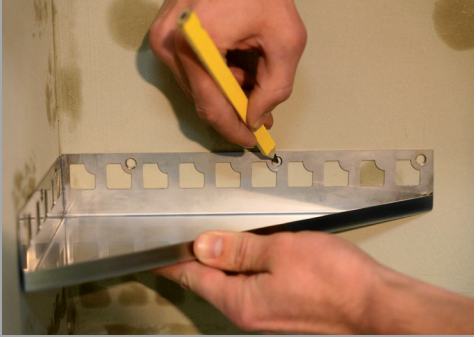
Bohrmarkierungen anzeichnen
