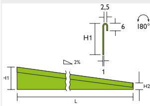
Schematische Darstellung Gefällekeil
